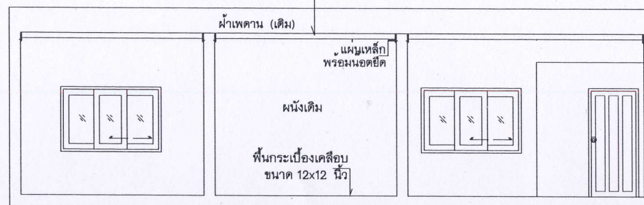
แบบรูปตัด 2 มาตราส่วน 1 : 50
