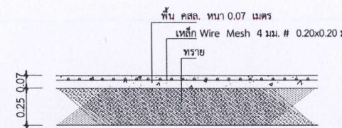
แบบรูปตัดพื้น คสล.
