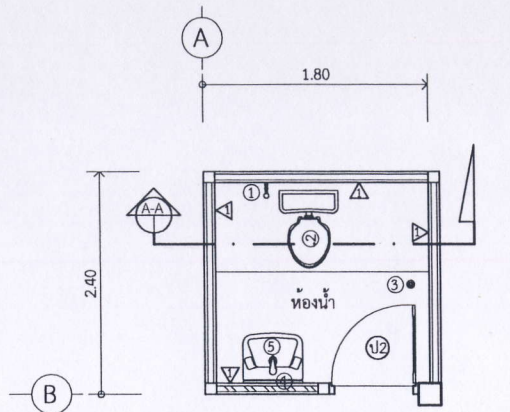
แบบขยายแปลนห้องน้ำ
